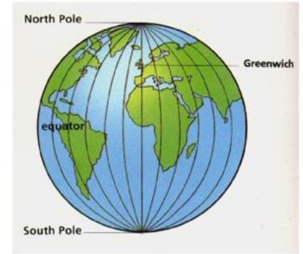
Lines of Longitude
